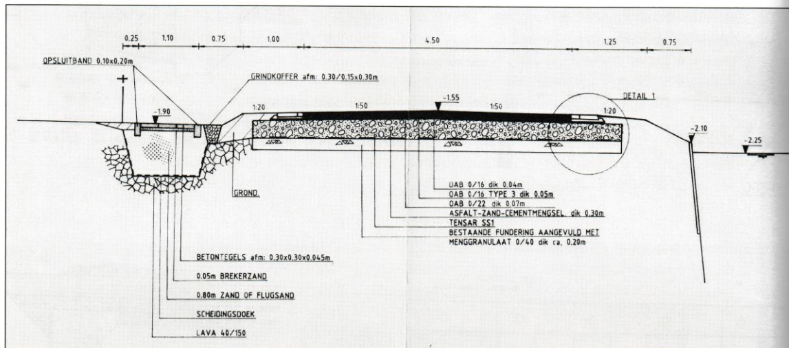
Dwarsprofiel van de 'Brugweg buiten de bebouwde kom' met links de te dempen noordelijke bermsloot
